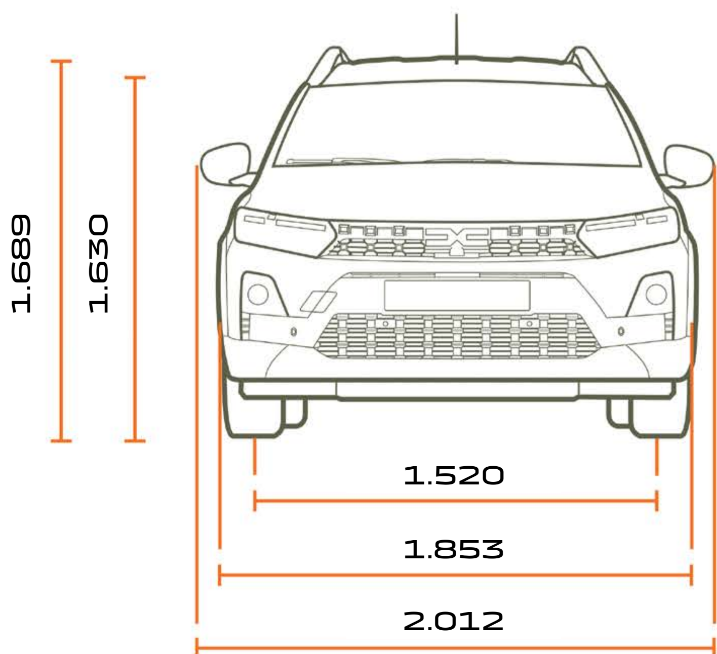
POGLED OD SPREDAJ VOZILA S 5 IN 7 SEDEŽI
