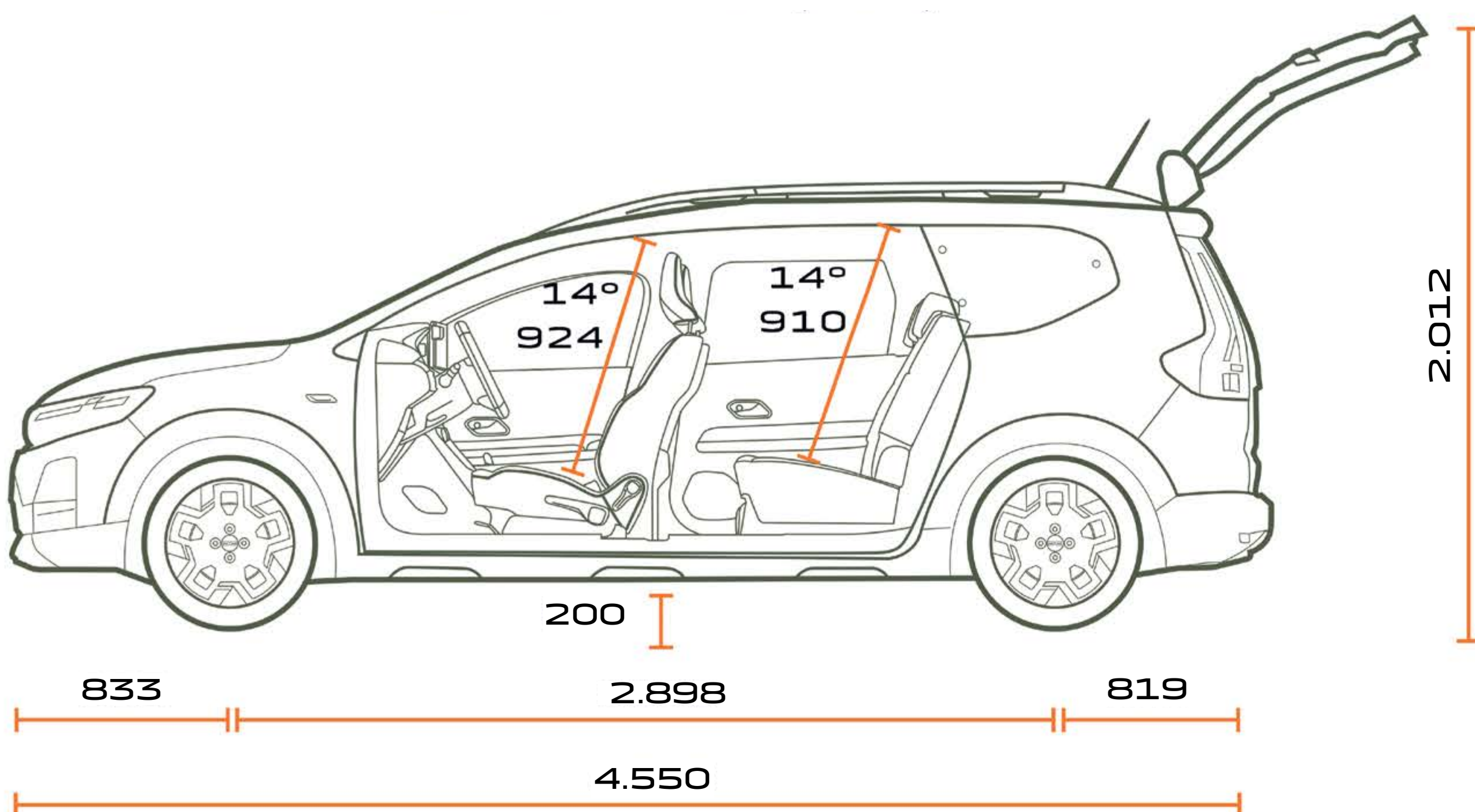
POGLED S STRANI VOZILA S 5 SEDEŽI
