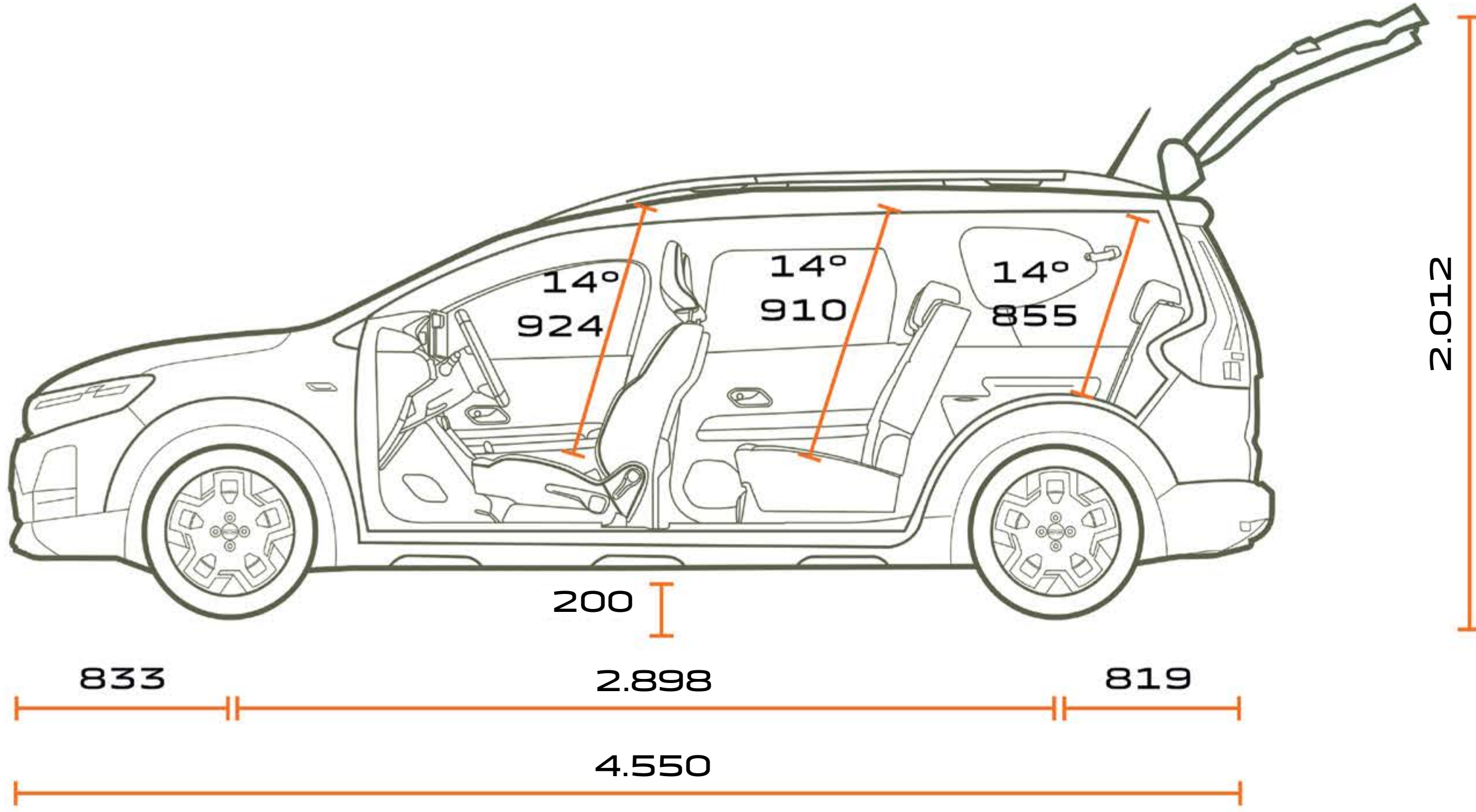
POGLED S STRANI VOZILA S 7 SEDEŽI
