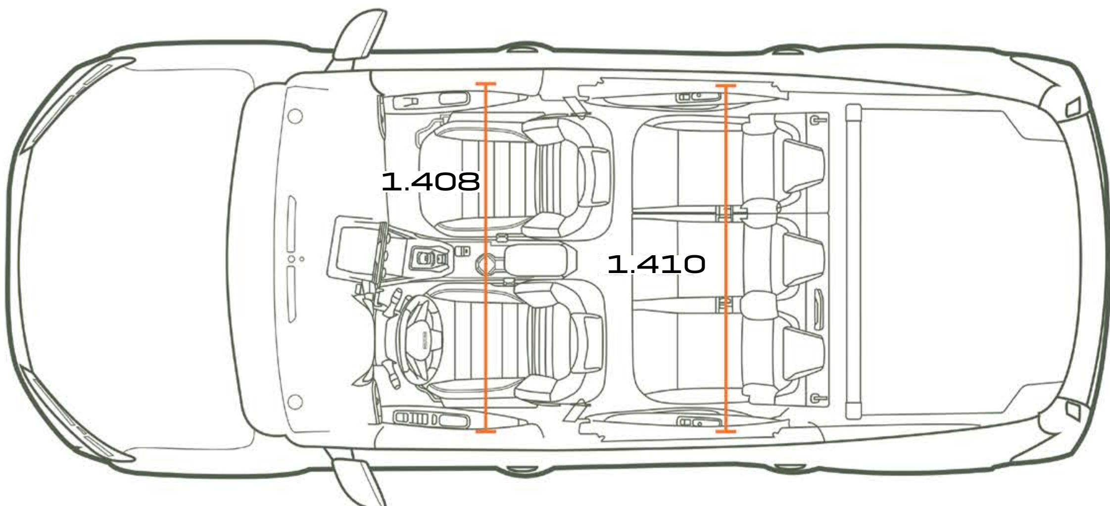
POGLED OD ZGORAJ VOZILA S 7 SEDEŽI
