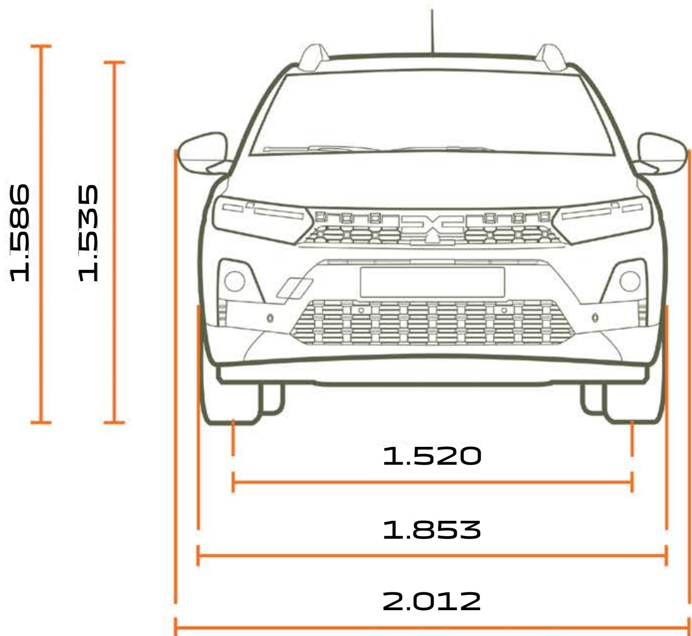
POGLED OD SPREDAJ
