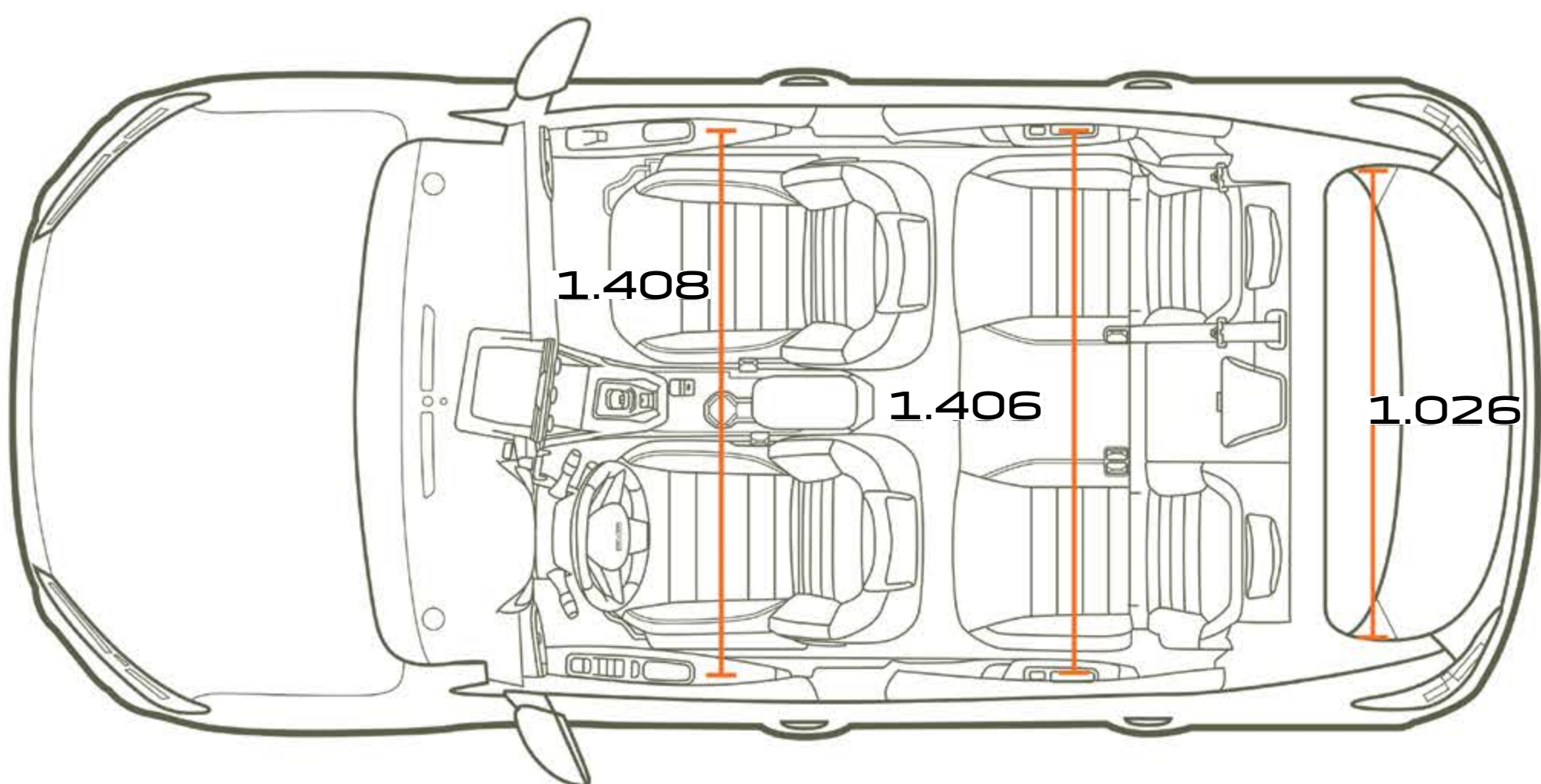
POGLED OD ZGORAJ
